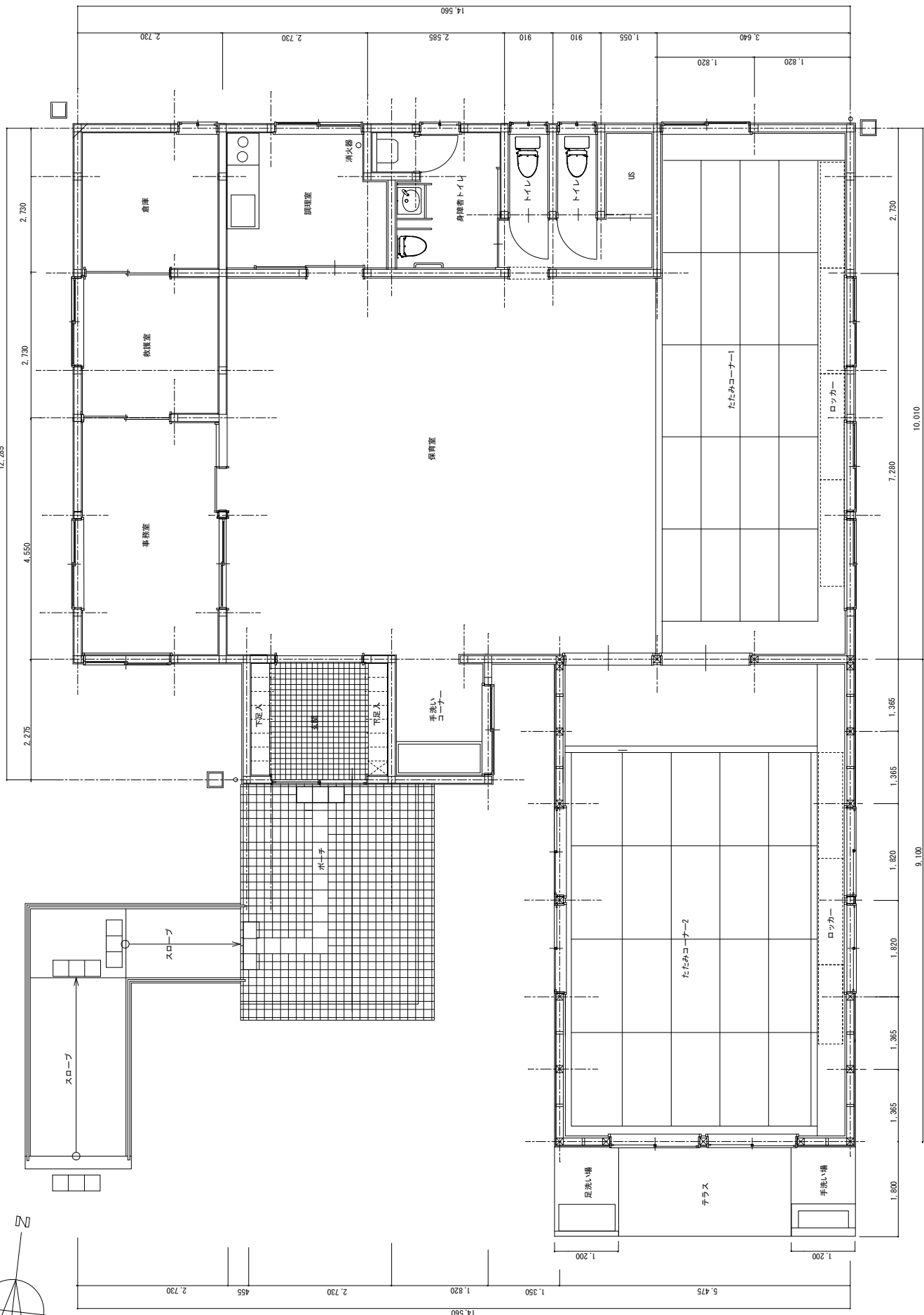
きらめきクラブいちのかわ平面図
