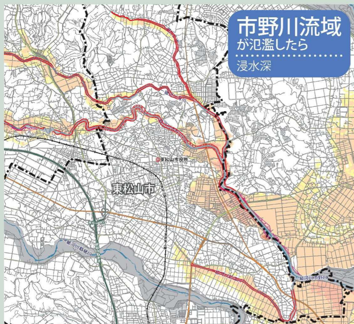
市野川流域洪水浸水想定区域図（想定最大規模）
